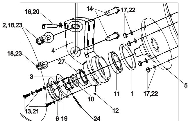
DETALLE A
